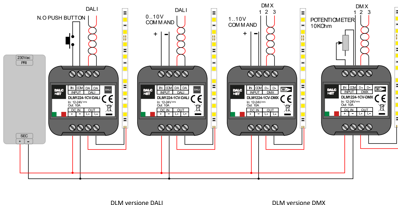
DLM versione DALI
